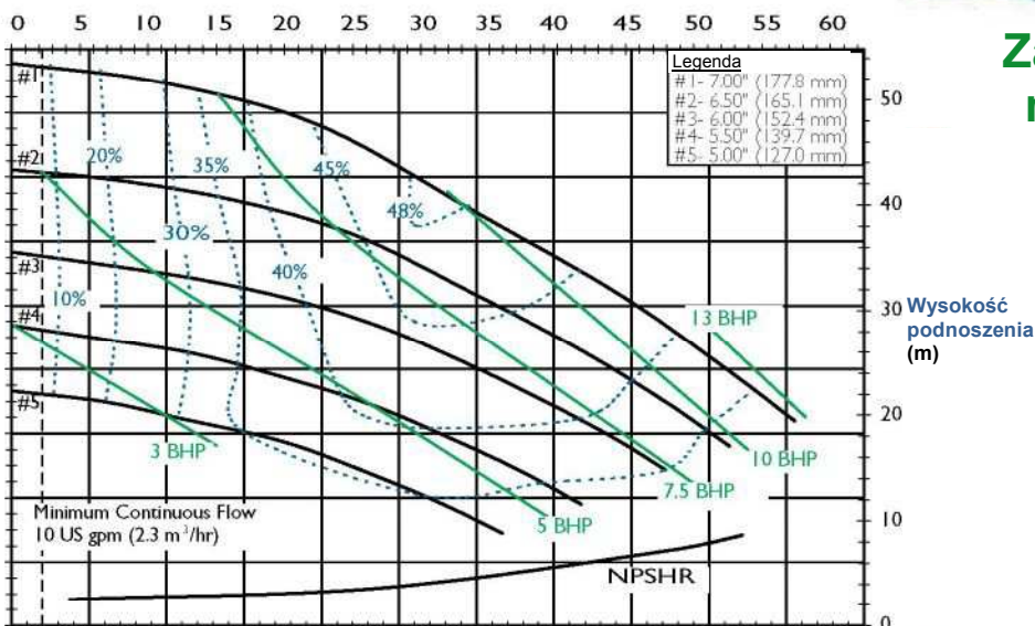
SP 22 WYDAJNOŚĆ przy wolnym napływie 2900 RPM
